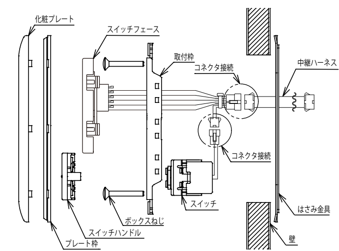
埋込表示スイッチ 組立・配線図
