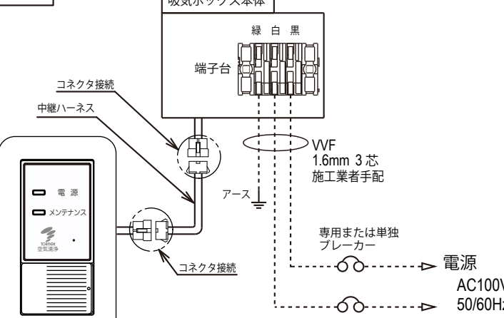
配線図
